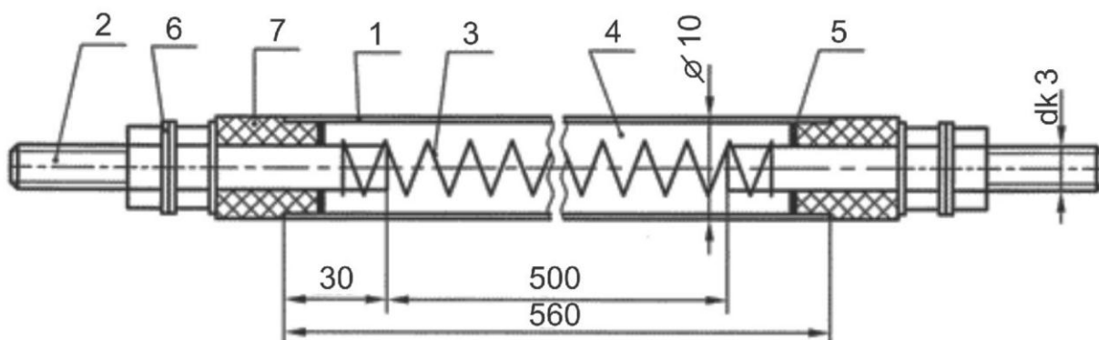
Конструкция ТЭНа (прямого).
